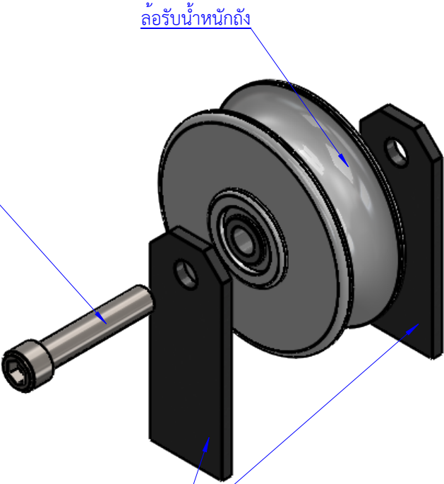
ชุดยึดล้อรองรับน้ำหนัก
