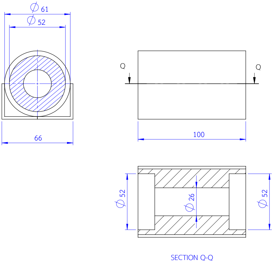
2.ชุดเสื่อลูกปืนรองรับเพลาคับ
